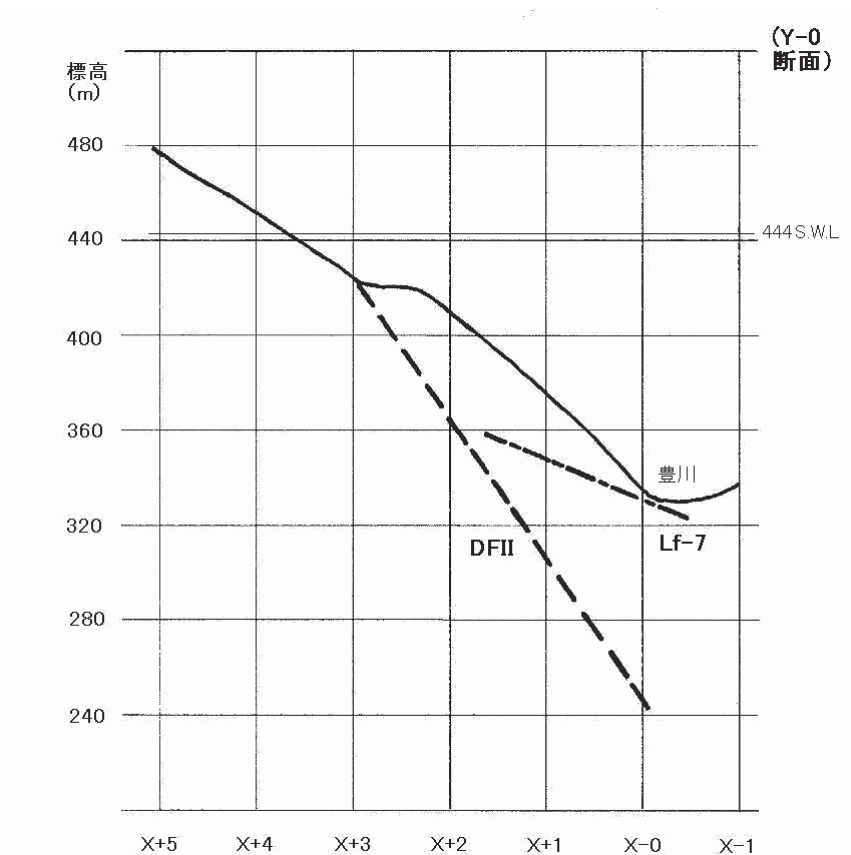
図-4 設楽ダムサイト計画地点左岸 (Y-0) 断面における断層
