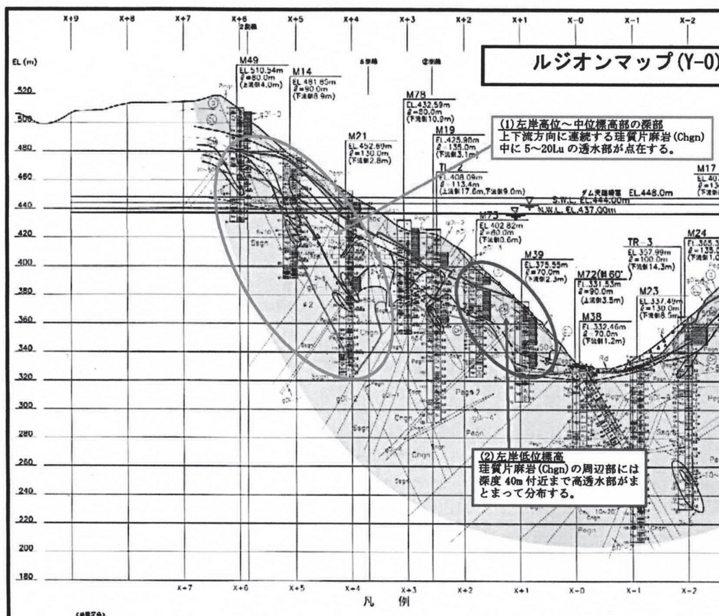
図-2 ダムサイト左岸の上下流（東西）方向に連なる二筋の高透水ゾーン、平成21年度設楽ダム地質総合解析業務報告書、図-9.1.4 Y-0ルジオンマップ（部分）
