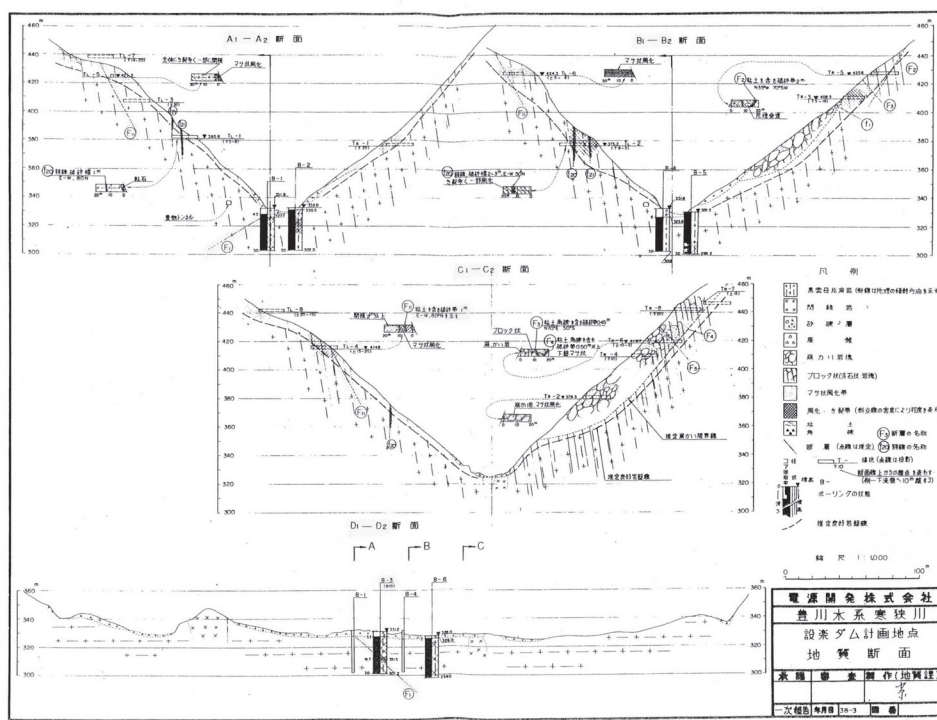
図-3b 設楽ダム計画地点地質断面 電源開発(株), 1963.3
