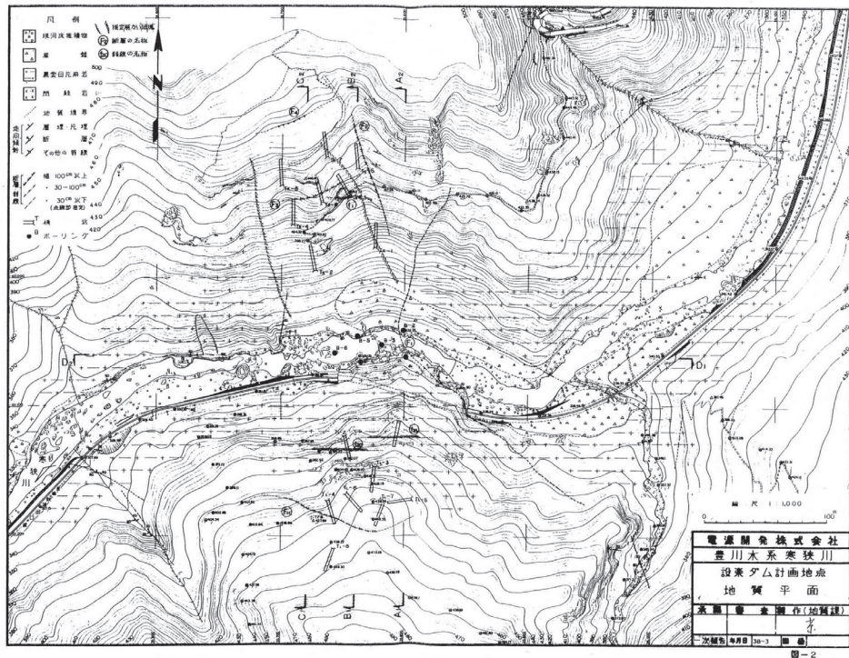
図-3a 設楽ダム計画地点地質平面 電源開発(株), 1963.3
